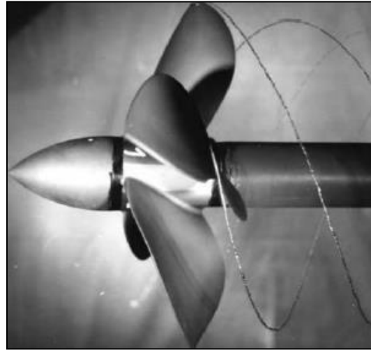
Fig. 6. Vortex cavitation
